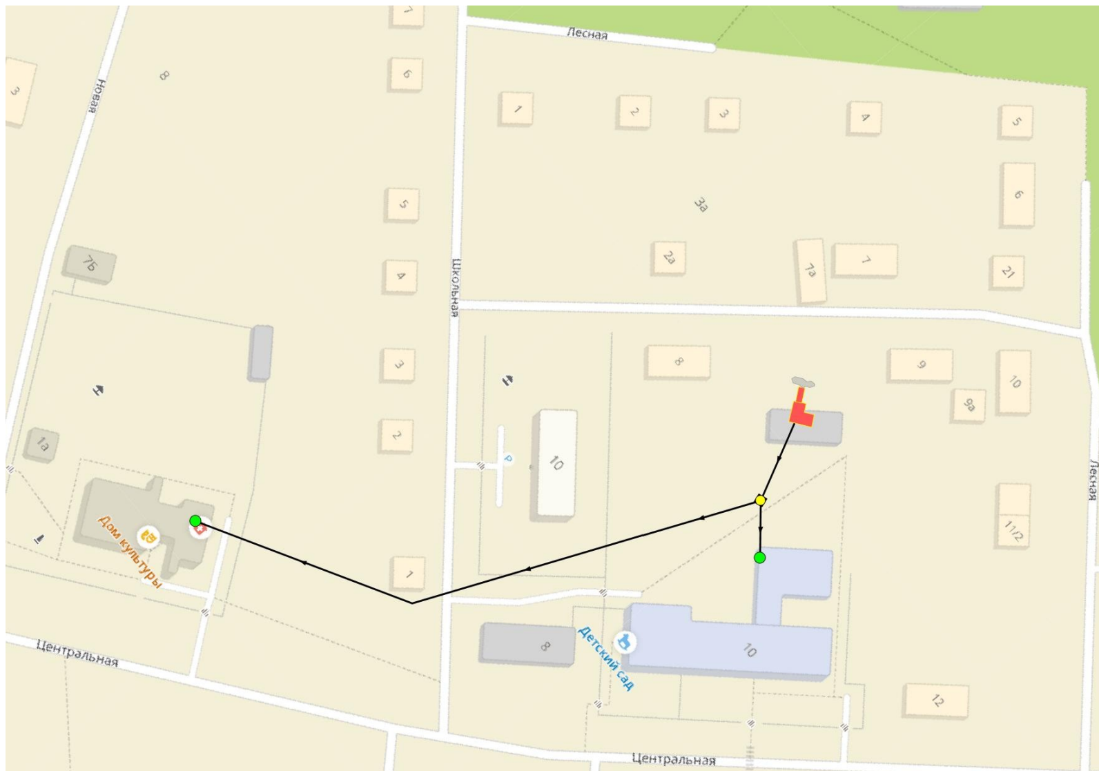
Рис. 2.1 Схема тепловых сетей котельной ЕТО АО «РПО «Таткоммунэнерго»
